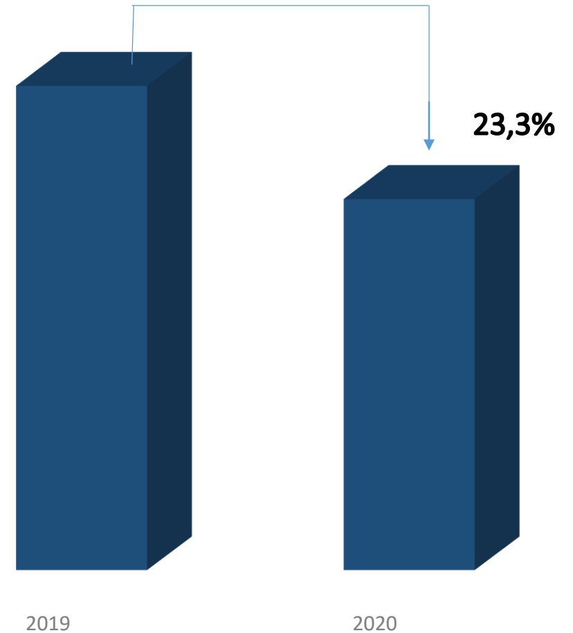
Ajrimlar dinamikasi
